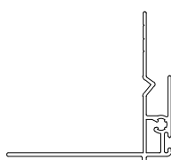
Alluminio 50 mm | 5451 listello per intonaco esterno
